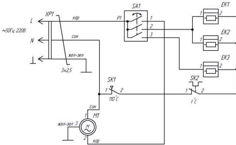
Схема коммутации переключателя SA1
